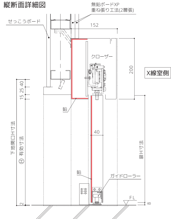
縦断面詳細図
